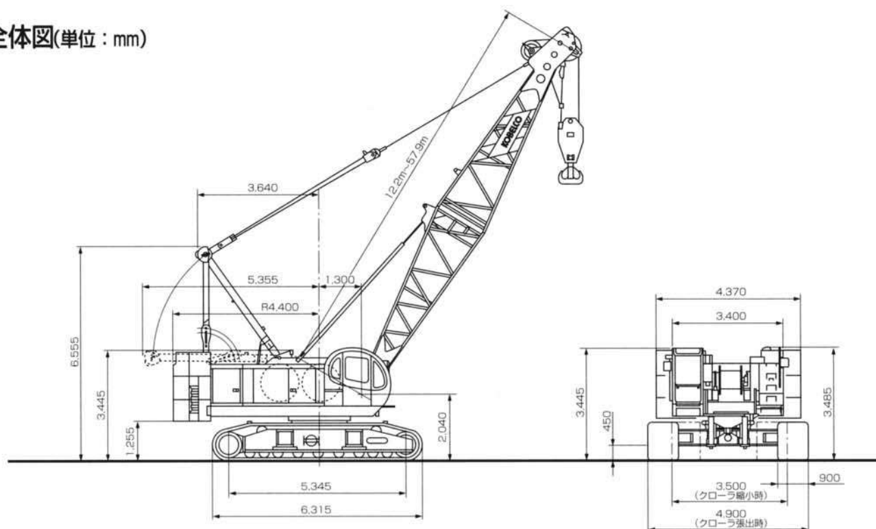
▶作動範囲図
